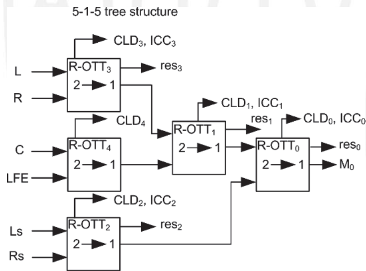
Fig. 4. OTT tree forming a 5.1-to-mono encoder.
